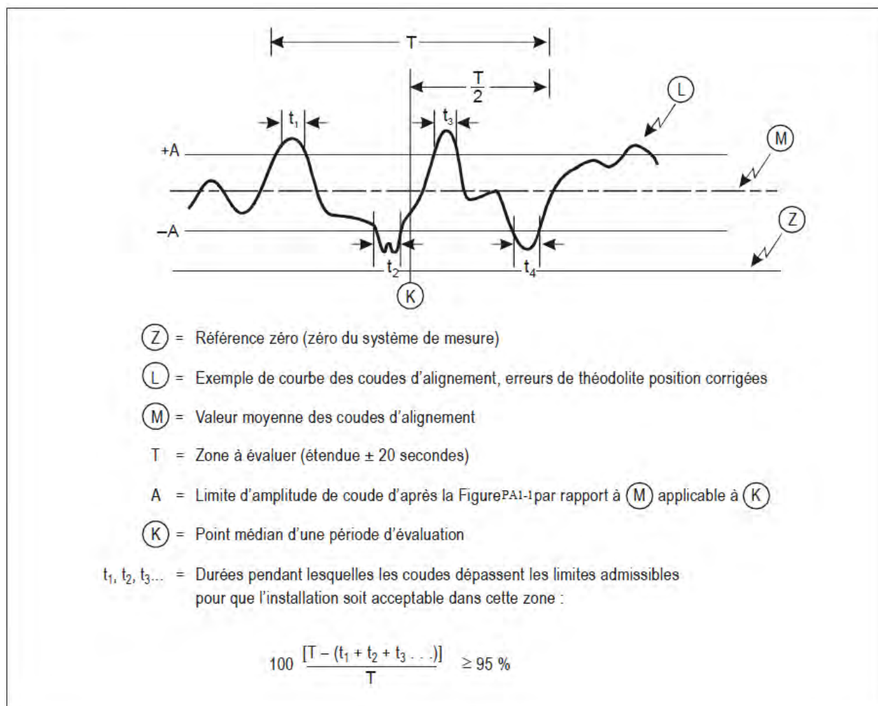
Figure C-2. Evaluation de l'amplitude des coudes d'alignement
