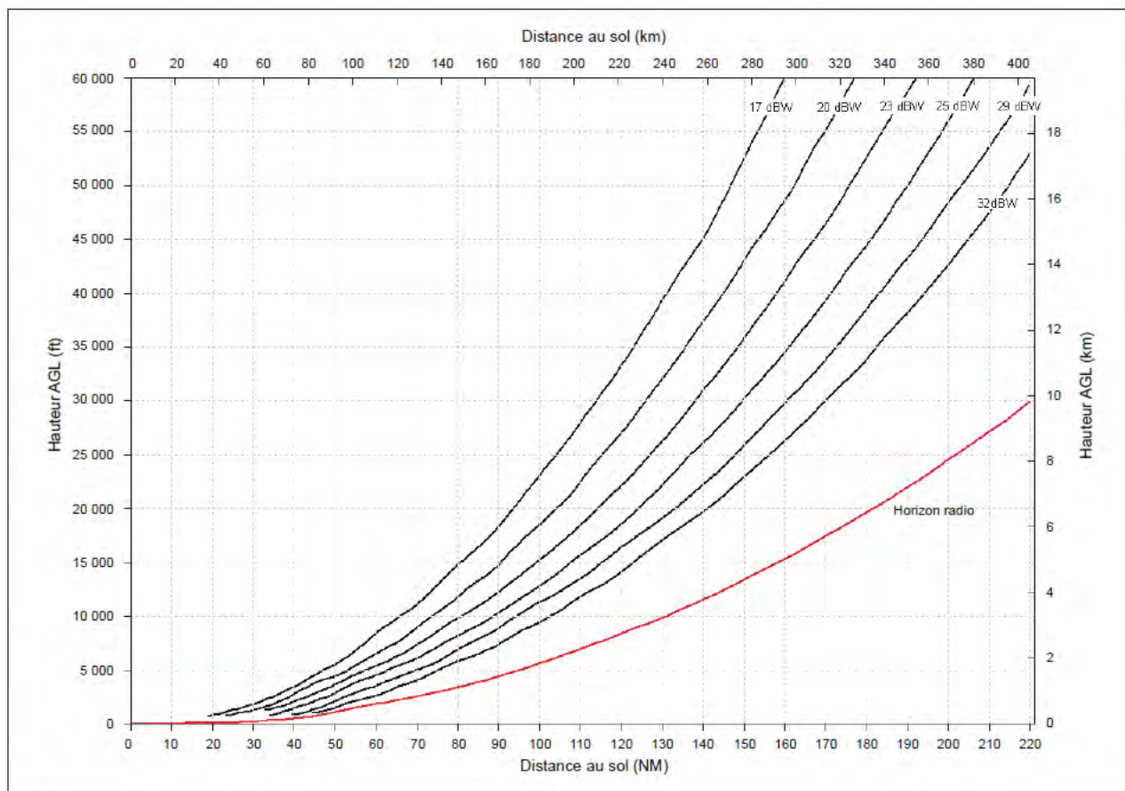
Figure C-13. P.i.r.e nécessaire pour obtenir une intensité de champ de 90 microvolts par mètre ( -107 \text{ dBW/m}^2 ) en fonction de la hauteur au-dessus du VOR/DVOR et de la distance par rapport au VOR/DVOR
