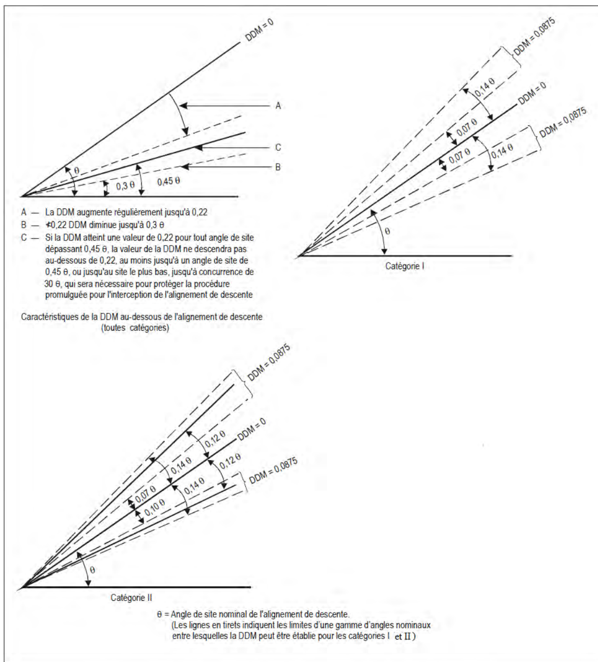
Figure C-11. Alignement de descente — Différence de modulation (DDM)
