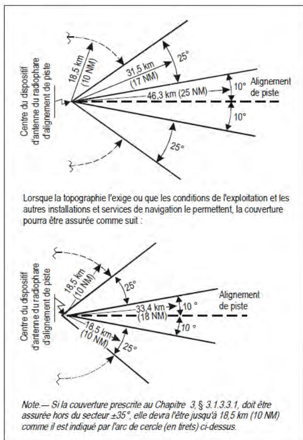
Figure C-7A. Couverture en azimut du radiophare d'alignement de piste
