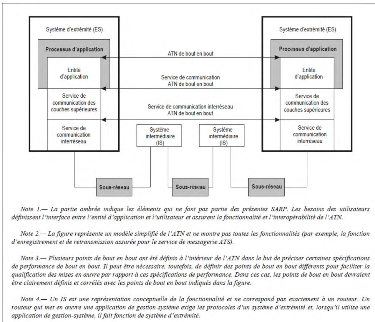
Figure 3-1. Modèle conceptuel de l'ATN
