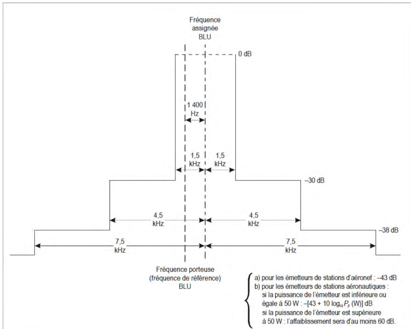
Figure 2-1. Limites du spectre requises (sous forme de puissance de crête) pour les émetteurs BLU de stations d'aéronef et pour les émetteurs BLU de stations aéronautiques
