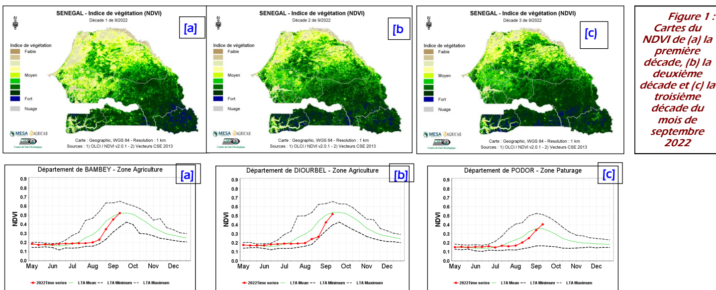
Figure 2 : Profil du NDVI à la troisième décade du mois de septembre 2022 des départements de (a) Bambeï, (2b) Diourbel, et (3) Podor (courbe rouge), en comparaison avec ceux des valeurs moyennes (courbe verte) et minimum et maximum (courbes discontinues noires) de la série historique 1999-2021
