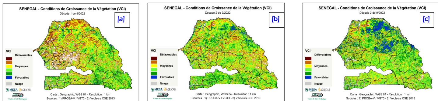
Figure 3 : Cartes du VCI de (a) la première décade, (b) la deuxième décade et (c) la troisième décade du mois de septembre 2022
