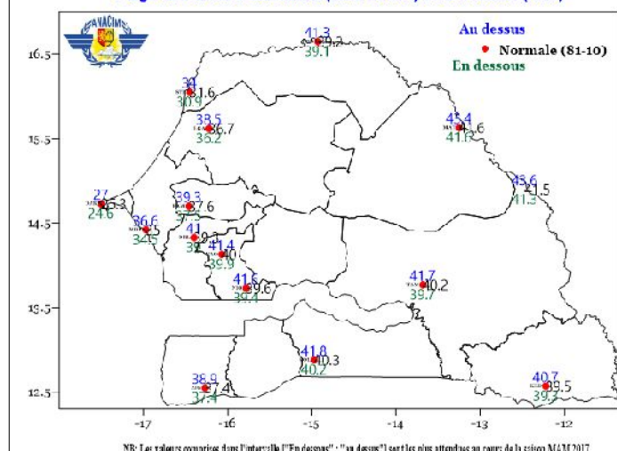
Prévision saisonnière des températures maximales au cours de la période Mars-Avril-Mai 2017 Plage des valeurs attendues (Bleu et vert) et la Normale (Noir)
