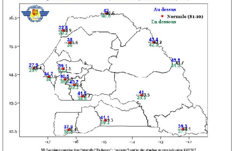
Prévision saisonnière des températures maximales au cours de la période Avril-Mai-Juin 2017 Plage de valeurs attendues (Bleu et vert) et la Normale (Noir)
